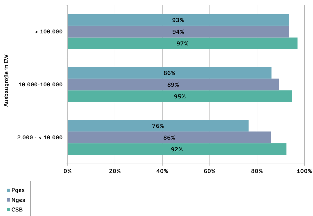
Abbildung 18: Prozentualer Frachtabbau für CSB, Nges und Pges der Kläranlagen >2.000 EW (gegliedert nach Grö- ßenklassen)
