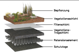
Detail- Schichtenaufbau
