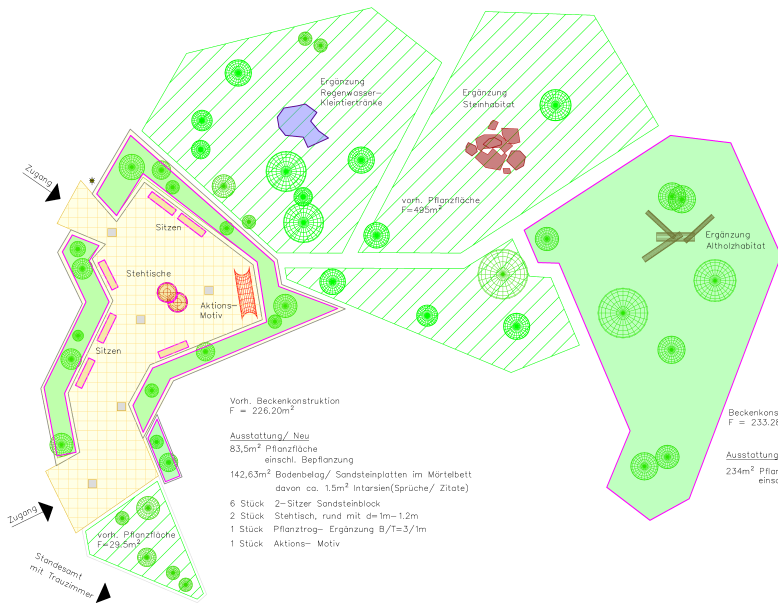
Lageplan-Wasserbecken/ Pflanzbeete
